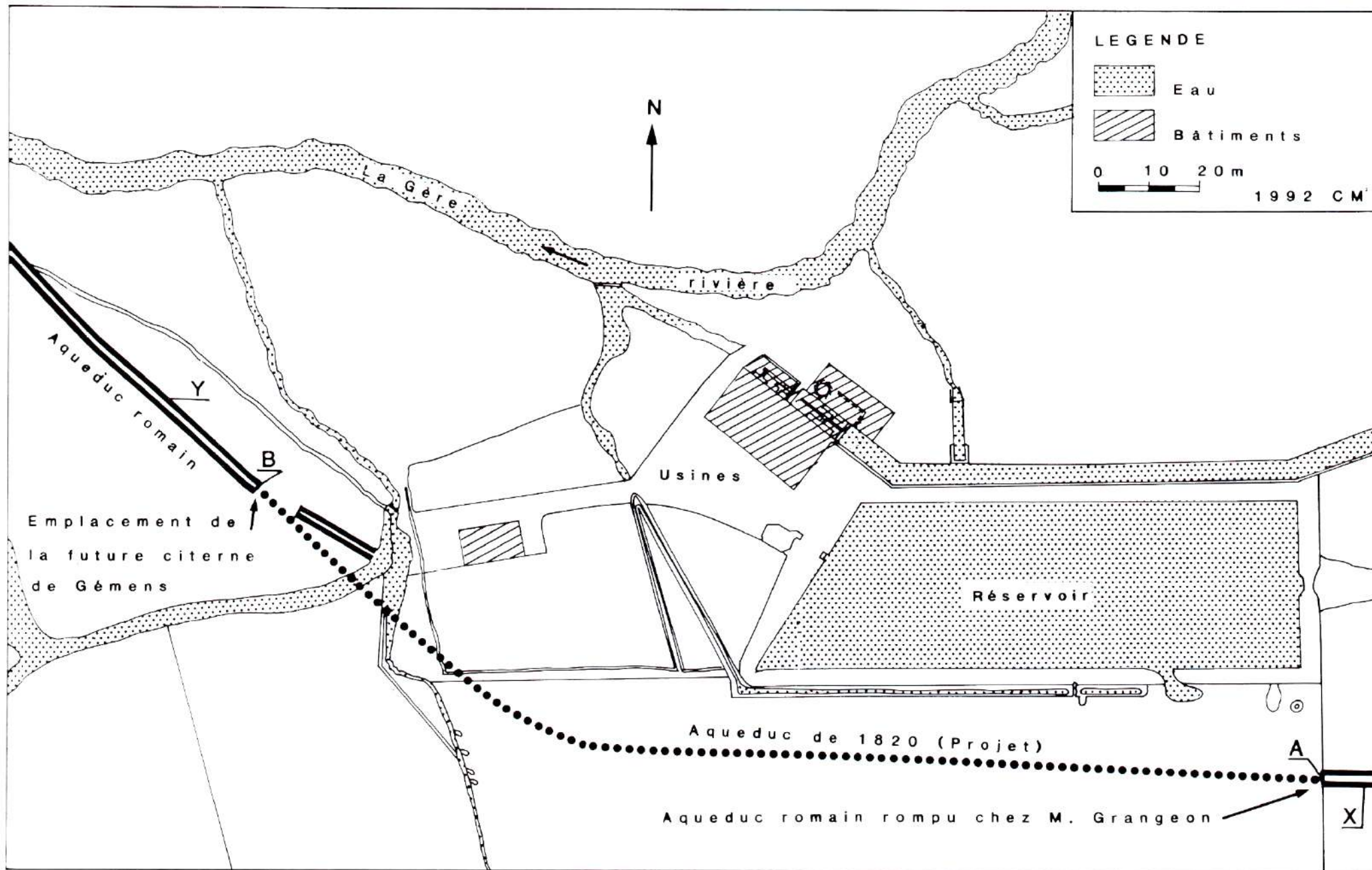
Fig. 2 : Plan du projet de construction de l'aqueduc de 1820 à Gémens, d'après le Plan des usines et propriétés environnantes appartenant à M. Grangeon (Estrablin) , par Elie Raymond, Avril 1820, 1/500 e , conservé aux Archives Municipales de la ville de Vienne, dossier M 12.
